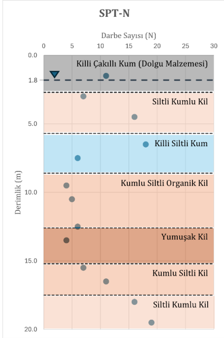
Şekil 2. Derinliğe bağlı SPT-N dağılımı (1 numaralı örnek sondaj)
