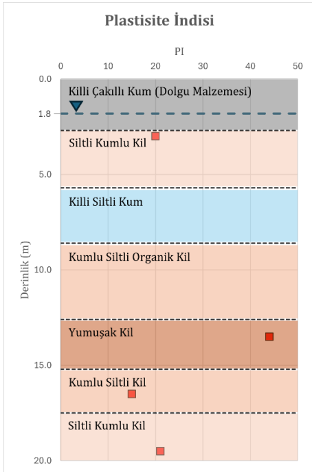
Şekil 4. Derinliğe bağlı PI dağılımı (1 numaralı örnek sondaj)
